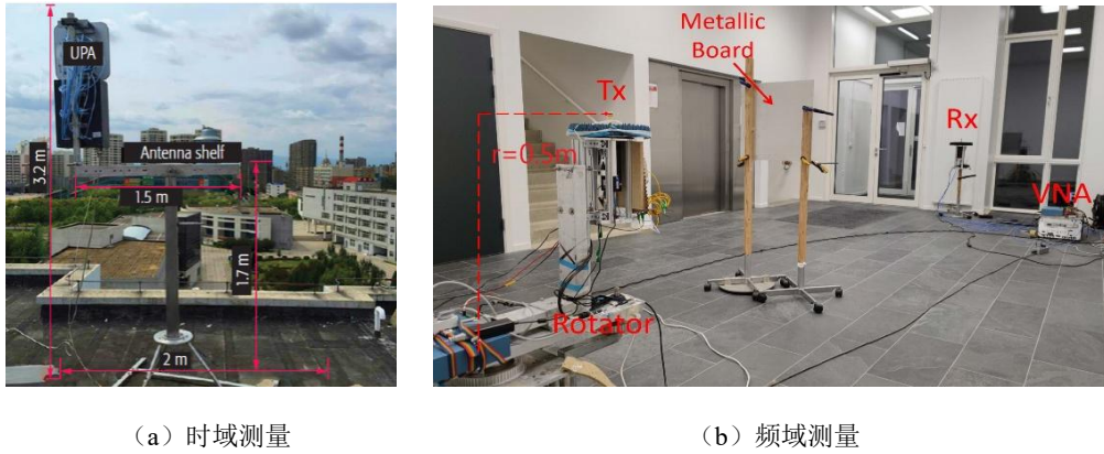
图 4.1 时域和频域的信道测量平台 [109][122]
