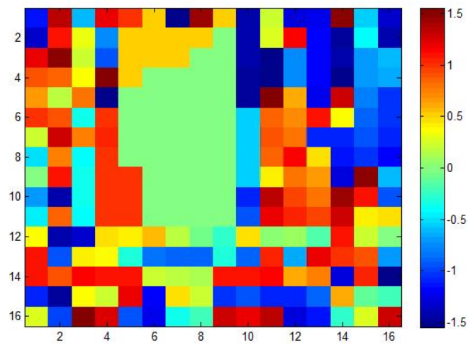
图 4.13 在基站阵列天线各单元阵子处 V 极化馈入波对应的信号强度增益分布
