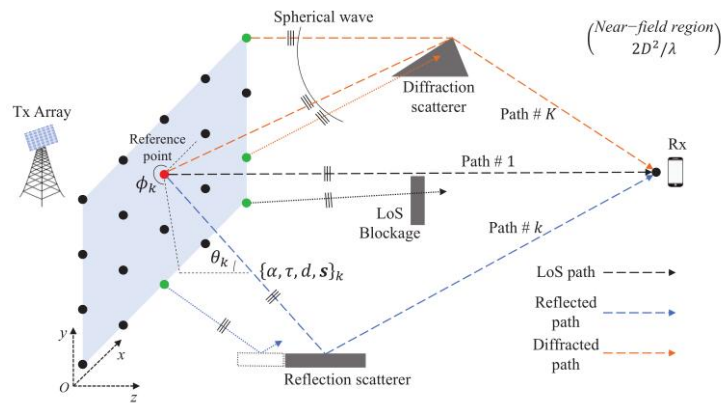
图 4.15 具有空间非平稳特性的近场球面传播
