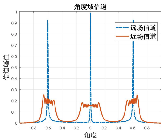
图 5.1 近场信道角度域能量扩散效应
