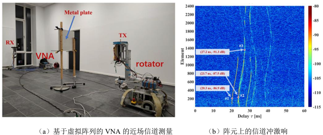
图 4.2 基于虚拟阵列的 VNA 的近场信道测量 [124]
