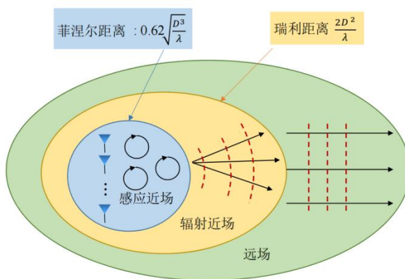
图 3.1 远场平面波面与近场球面波面及对应物理空间归一化接收能量
