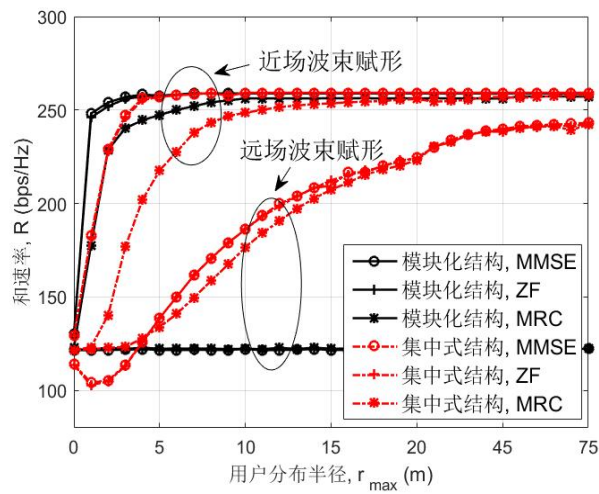
图 3.16 模块化和集中式 ELAA 可达和速率随用户分布半径变化关系 [92]
