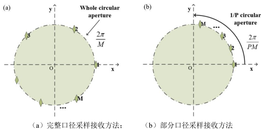
图 6.24 完整口径采样接收方法与部分口径采样接收方法示意图 [249]
