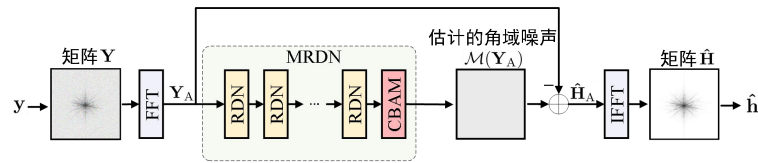
图 5.4 基于 MRDN 的信道估计方案
