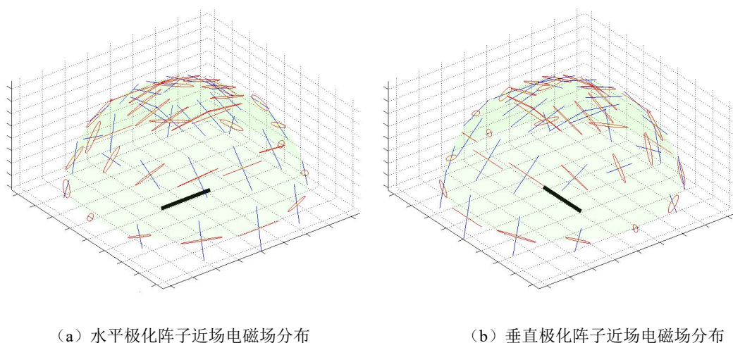
图 4.3 收发天线单元之间为近场时阵子近场电磁场分布的仿真结果
