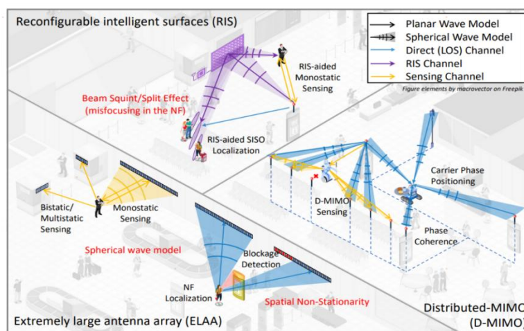
图 2.9 近场定位示意图
