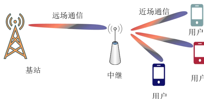
图 5.22 基于近场中继的混合通信架构
