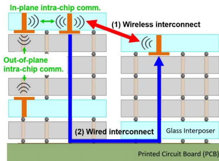
图 6.33 三维封装系统(SiP)中利用玻璃通孔(TGV)集成天线的面内/面外/片内/片间无线通信
