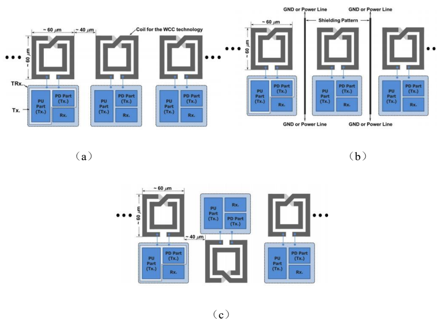
（a）传统电感线圈耦合阵列 （b）插入屏蔽结构 （c）之字形结构
