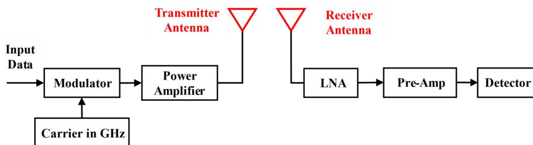
图 6.28 常用的片上通信系统框图 [252]
