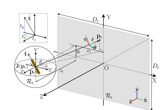
图 6.2 近场定位与姿态感知系统图
