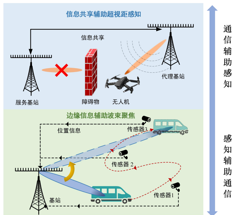
图 6.13 通信辅助近场感知和感与辅助近场通信示意图
