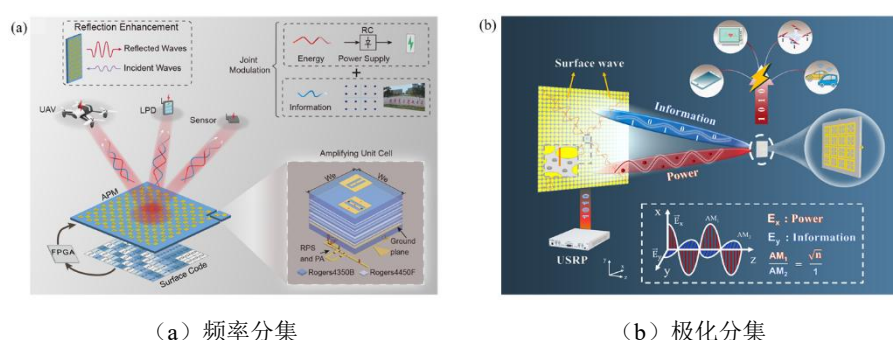
图 6.19 基于频率分集和极化分集的携能通信系统
