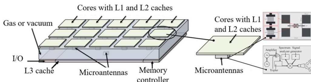
图 2.15 使用片上无线通信技术的单片多核处理器
