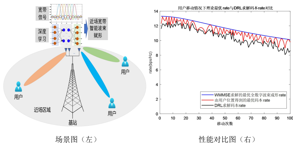
图 6.27 近场宽带智能波束赋形
