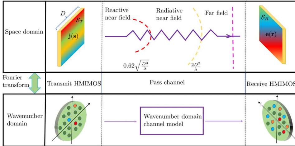
图 3.20 傅立叶平面波展开信道建模
