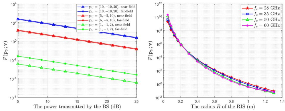
图 3.19 HRIS 辅助定位性能
